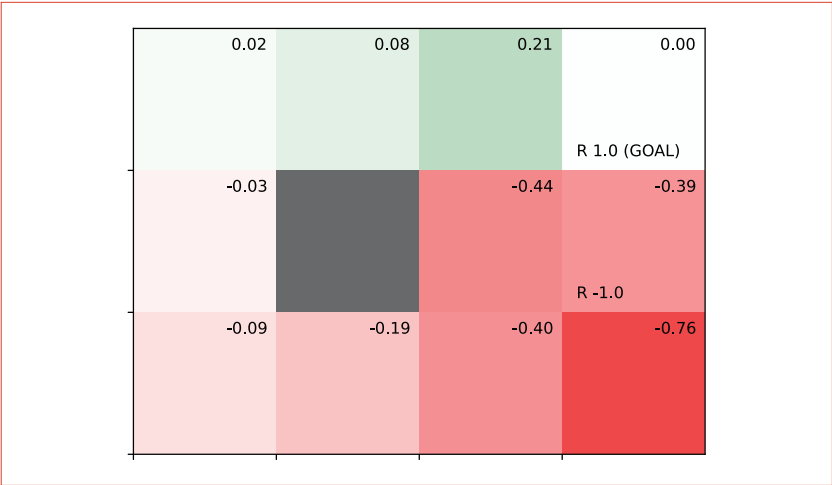
图 5-12 通过蒙特卡洛方法得到的价值函数
